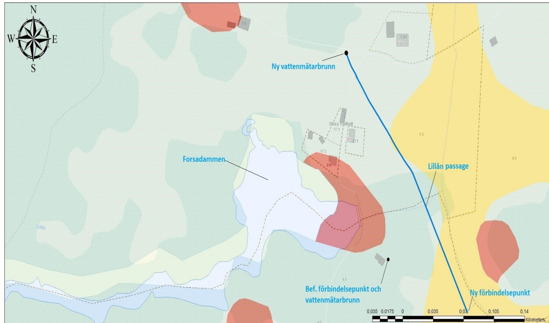
Alternativ förlägga vattenledning på land (blått streck = ny sträcka för vattenledning)
